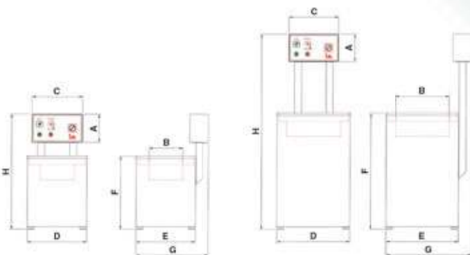
MOD. 500 ECO
