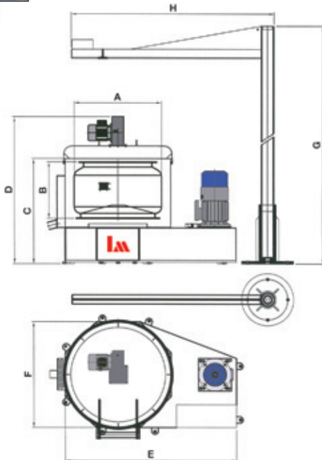
Cesto in acciaio inox AISI 304. Stainless steel basket AISI 304.
